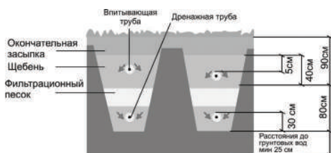
Рис. 6 Поперечное сечение фильтрационной площадки
