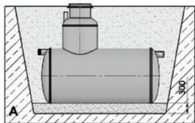
Рис. 3 Схема монтажа
